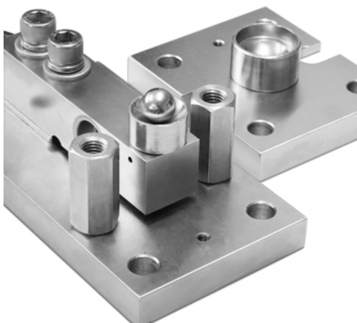
Dettaglio dello snodo sferico centrale a sfera
