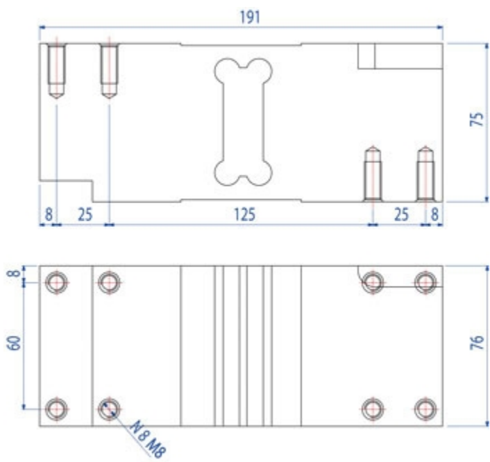
Dimensioni (mm)
